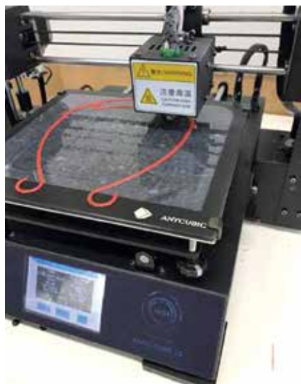
企業が保有する3Dプリンターでフェイスシールドのフレームを製作
